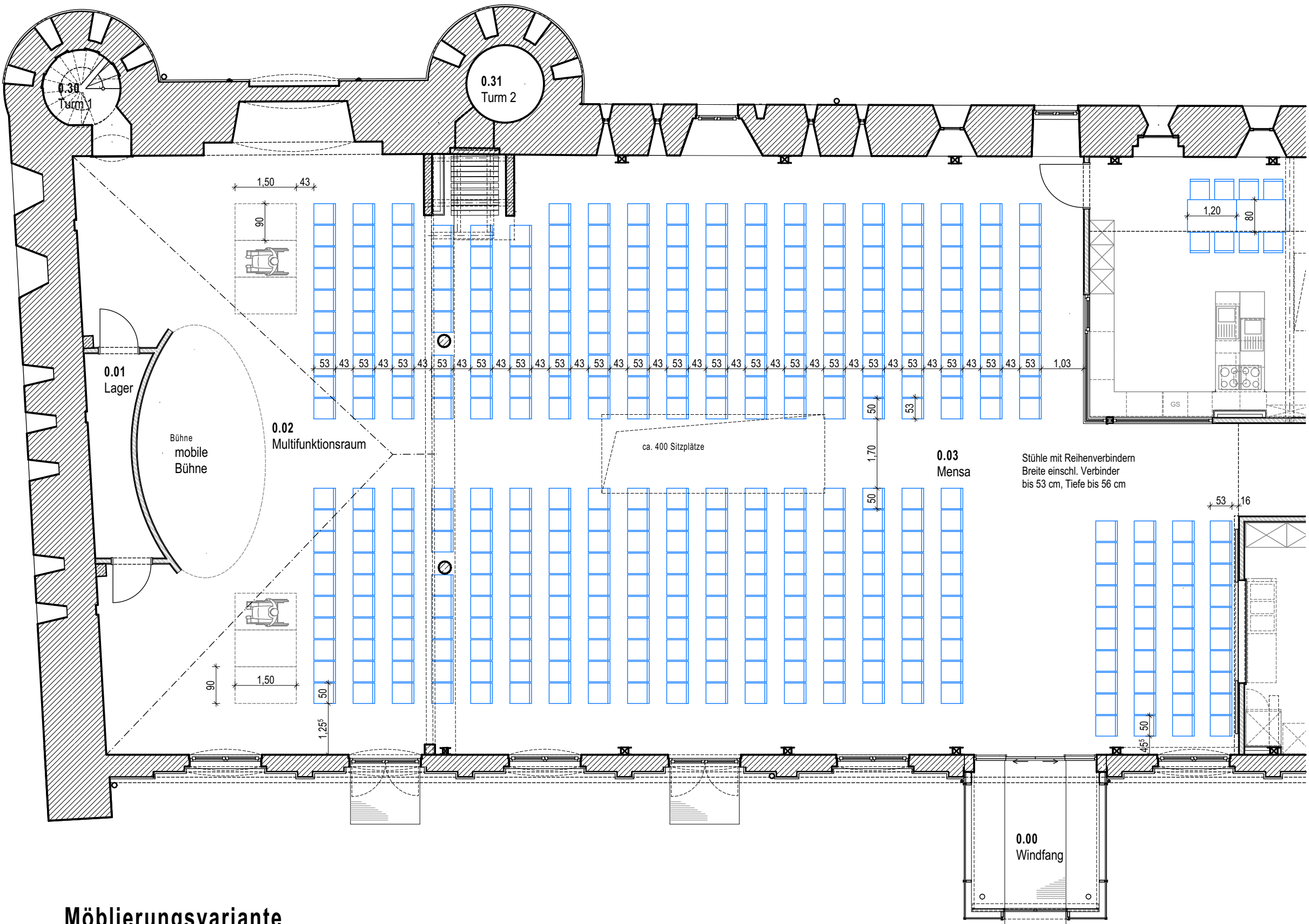
Möblierungsvariante "Reihenbestuhlung"
